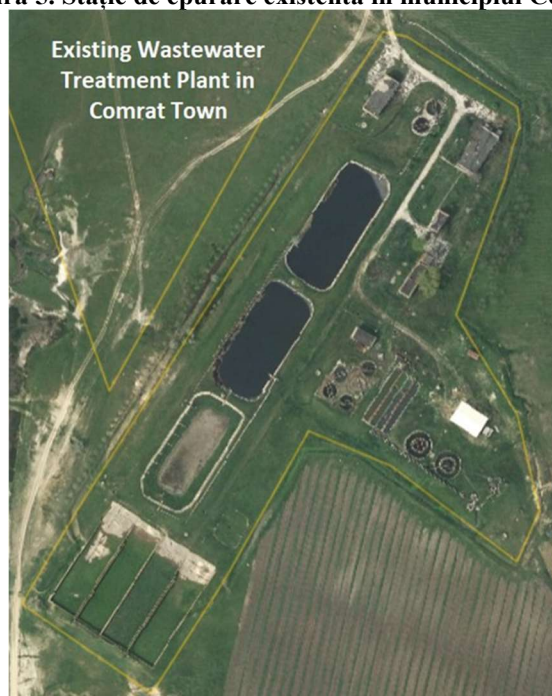
Figura 5. Stație de epurare existentă în municipiul Comrat
