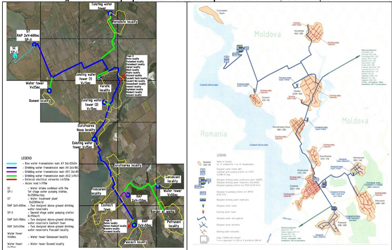
Figura 3. Schema propusă de alimentare cu apă în clusterul Prut, raionul Rîșcani
