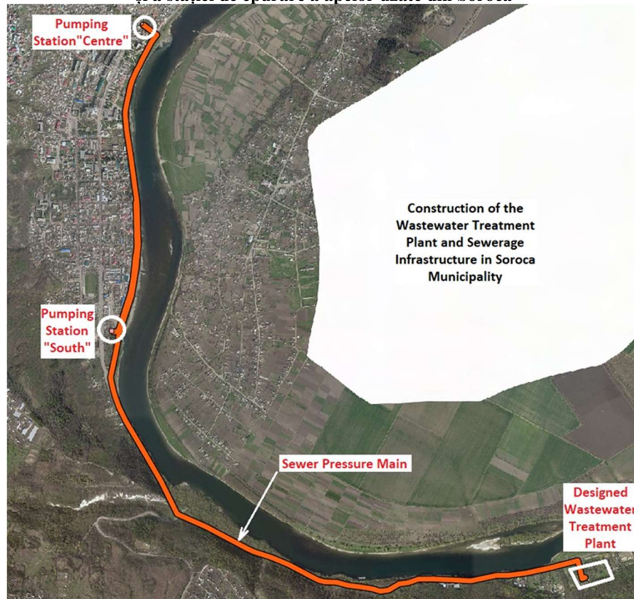
Figura 4. Planul rețelelor de canalizare sub presiune, a stațiilor de pompare și a stației de epurare a apelor uzate din Soroca
